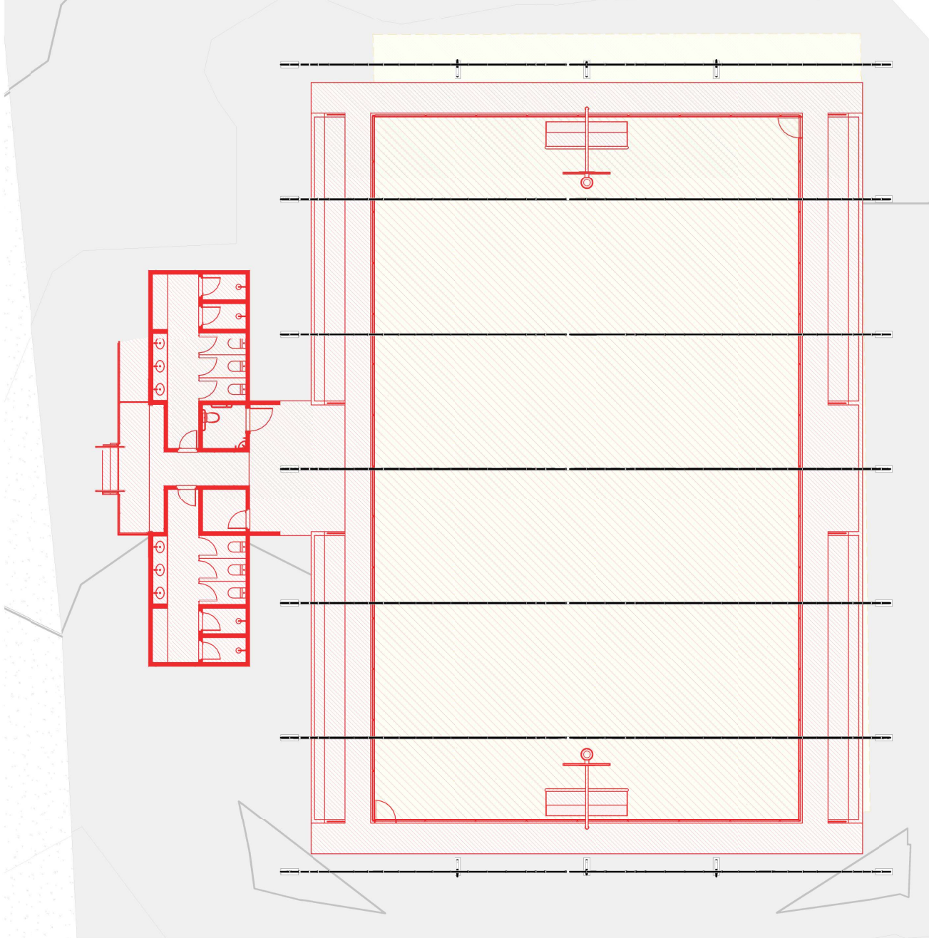
1 | PLANTA BAIXA - CONSTRUIR / DEMOLIR 1:75
