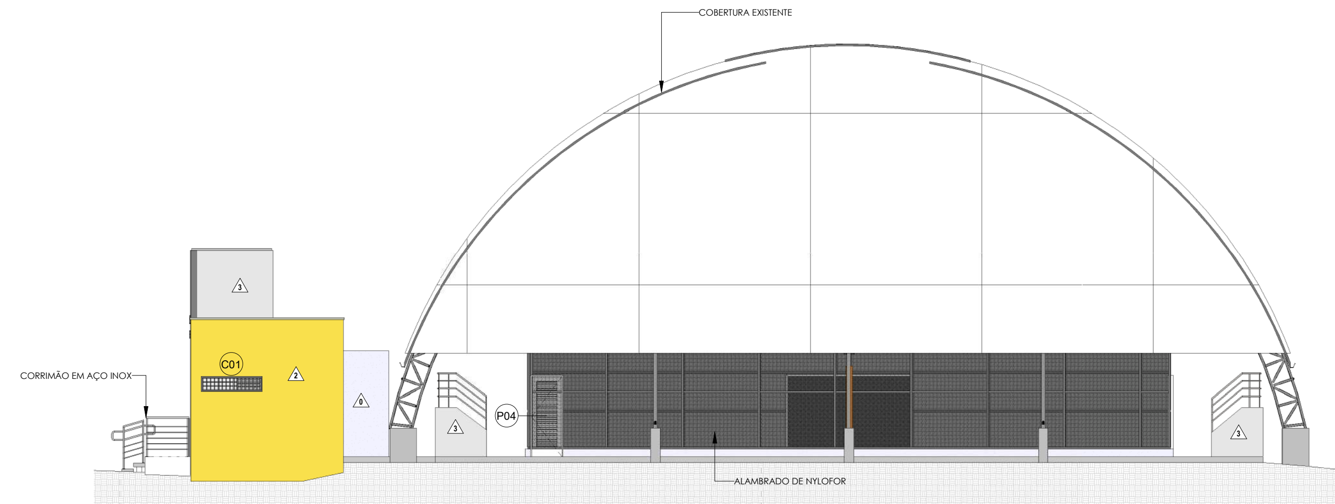
2 FACHADA LATERAL 1 1 : 100
