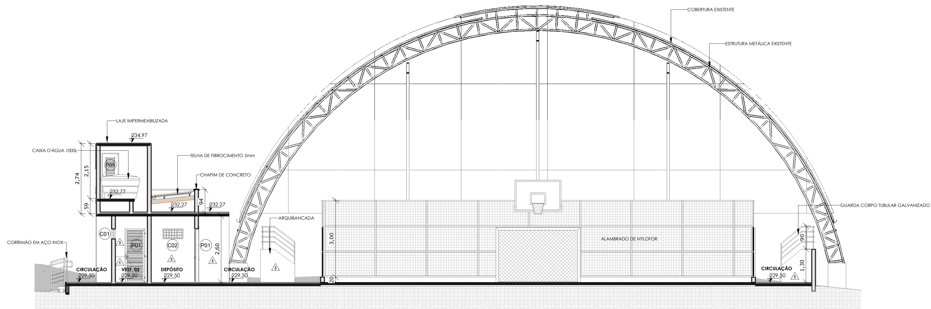
2 | CORTE 02 1:75
