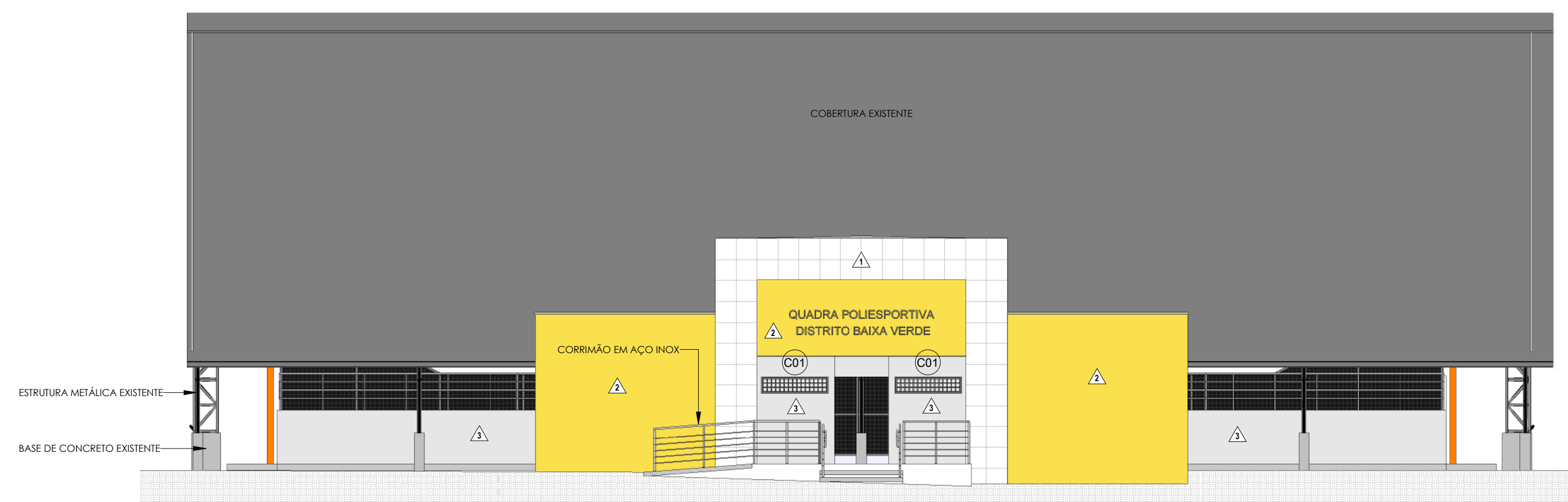
1 FACHADA FRONTAL 1 : 100
