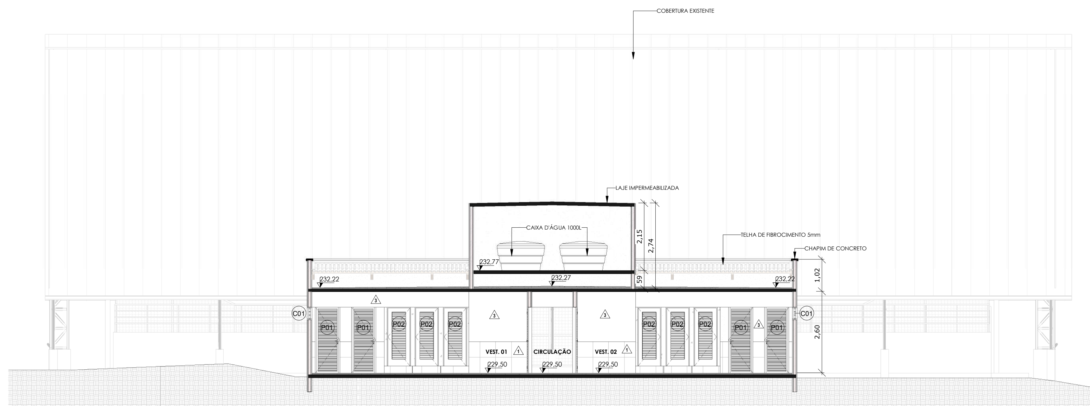
1 | CORTE 01 1:75
