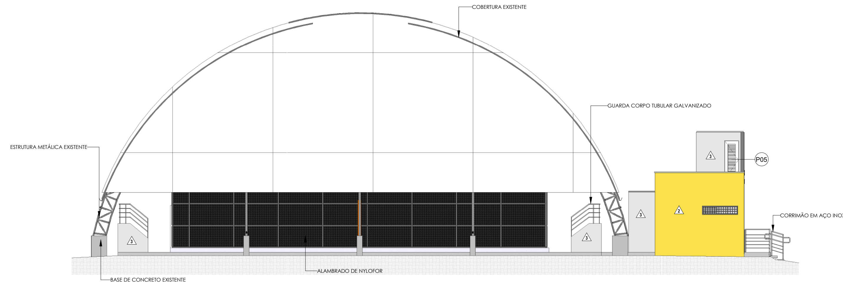
3 FACHADA LATERAL 2 1 : 100
