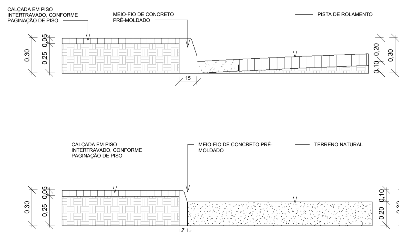
DET. MEIO-FIO 1 : 20
