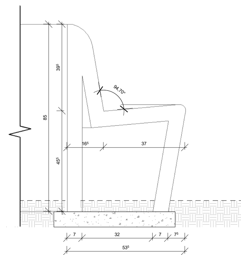
8 | CORTE - Banco de Concreto Curvo 03 1 : 10
