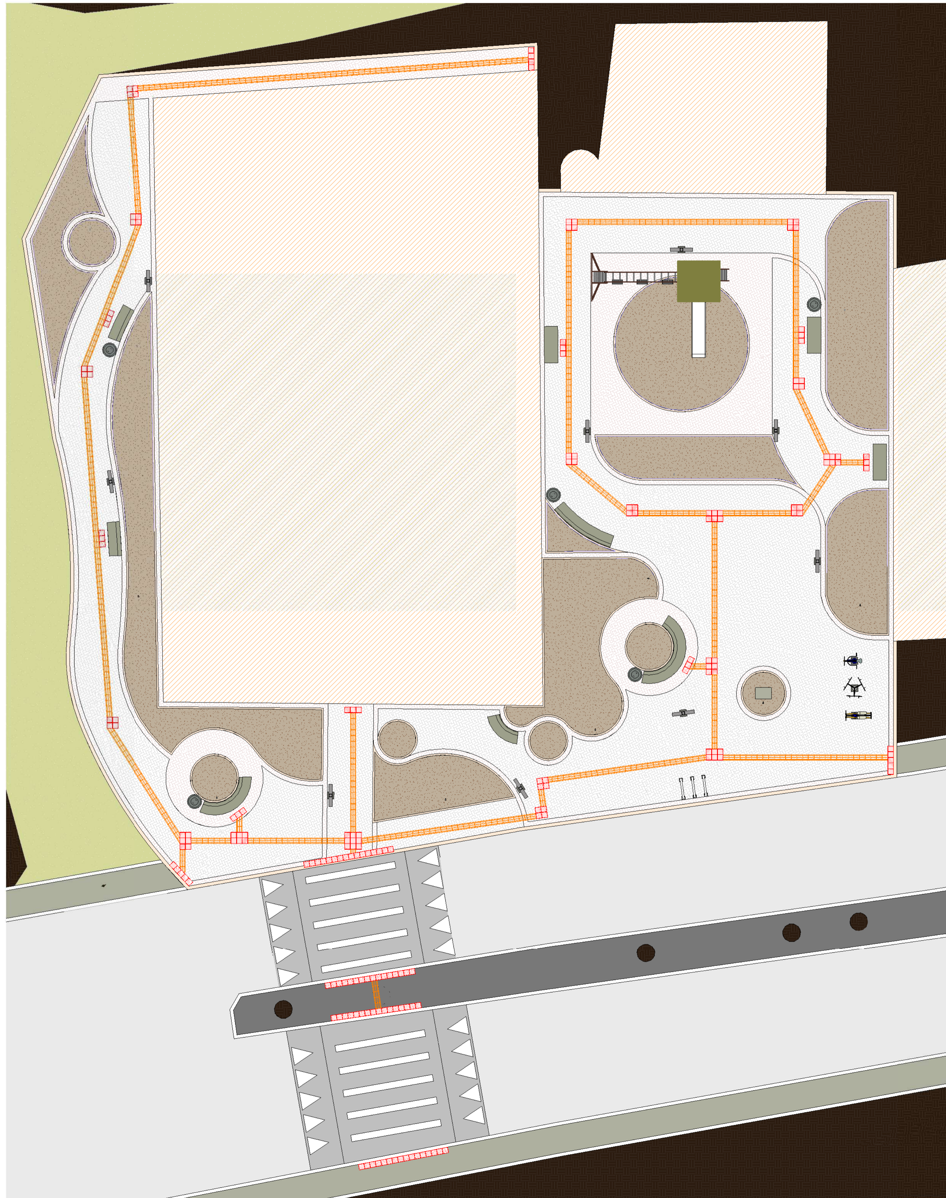
1 | PLANTA DE ACESSIBILIDADE 1:100
