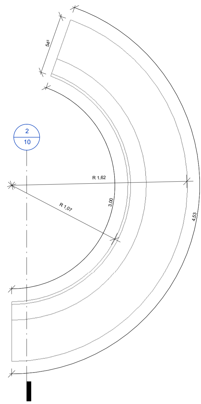
1 | PLANTA BAIXA - Banco de Concreto Curvo 01 1 : 20
