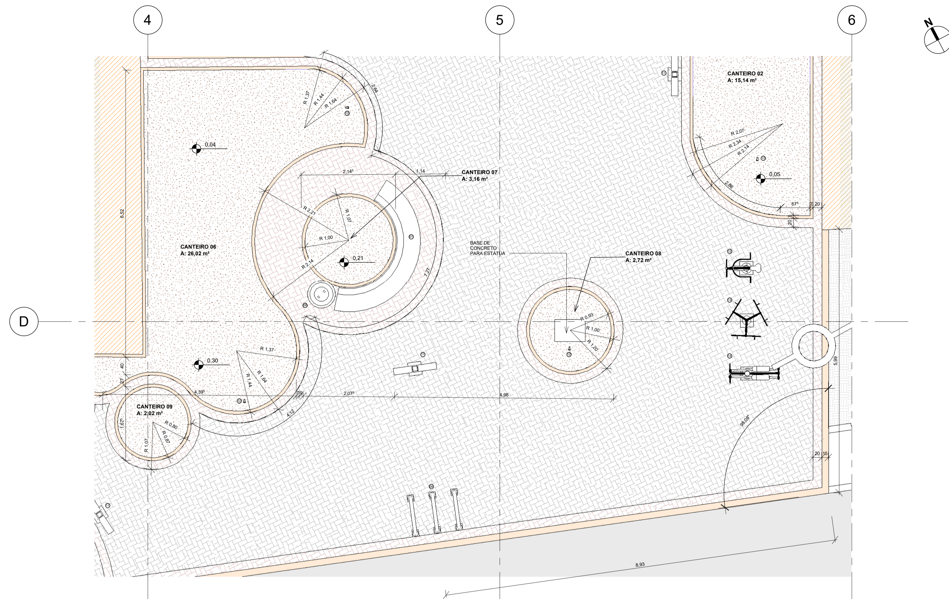
2 | PLANTA BAIXA - AMPLIAÇÃO TRECHO 04 1 : 50
