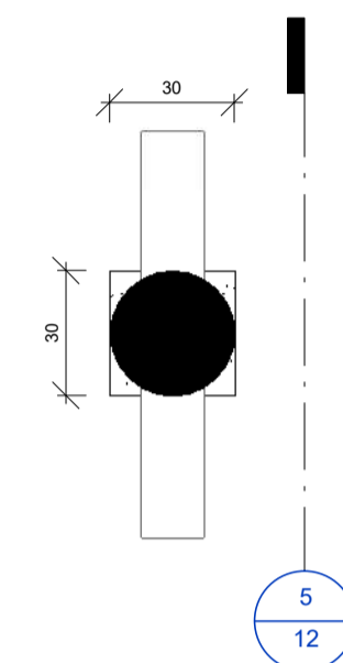
4 | PLANTA BAIXA - Poste de Iluminação 1 : 20
