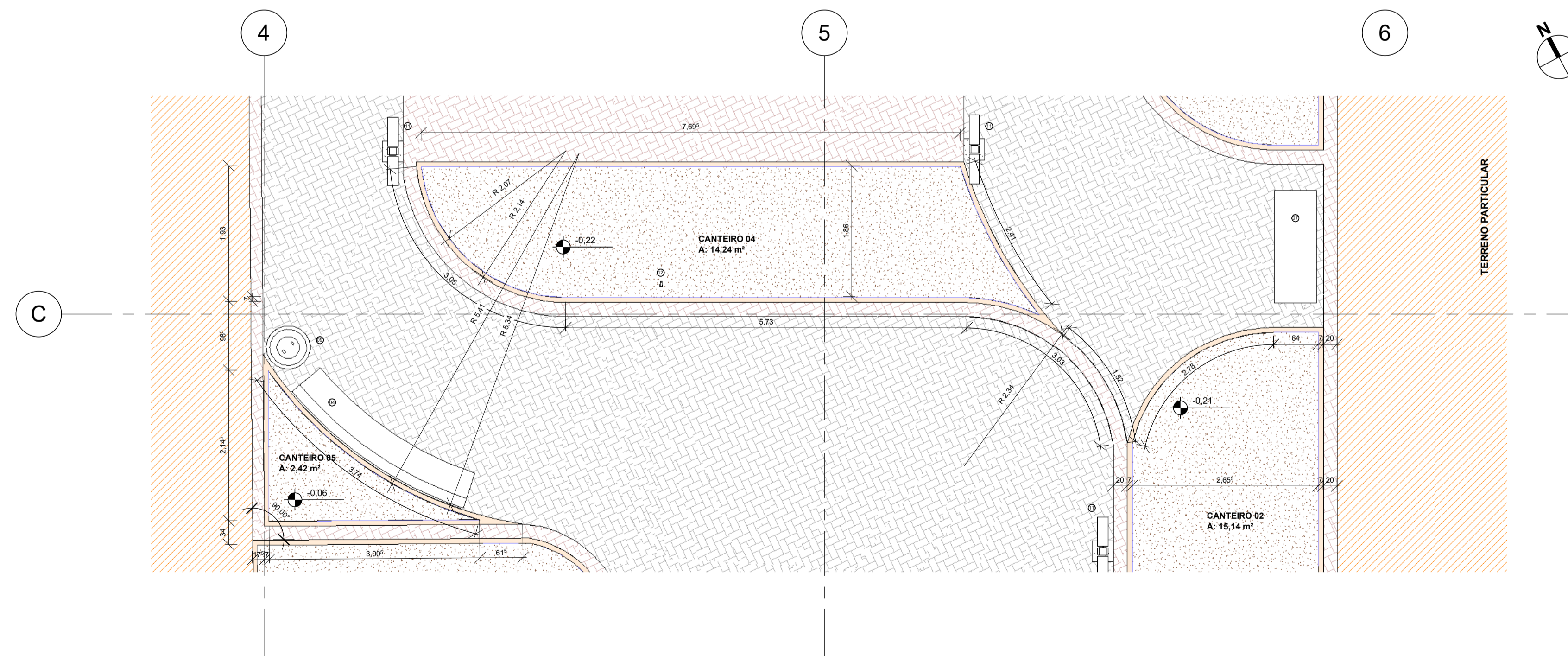
1 | PLANTA BAIXA - AMPLIAÇÃO TRECHO 05 1:50
