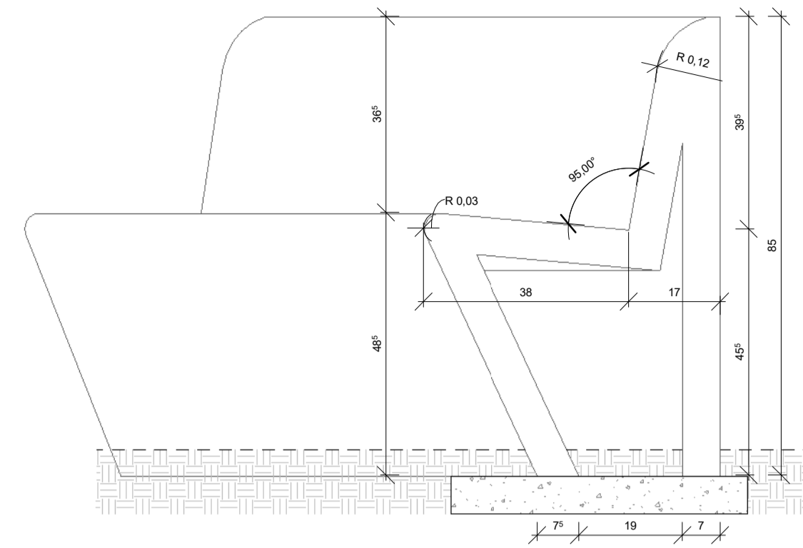
2 | CORTE - Banco de Concreto Curvo 04 1:10
