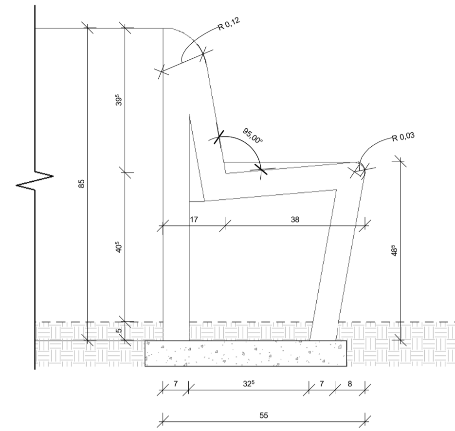
2 | CORTE - Banco de Concreto Curvo 01 1 : 10
