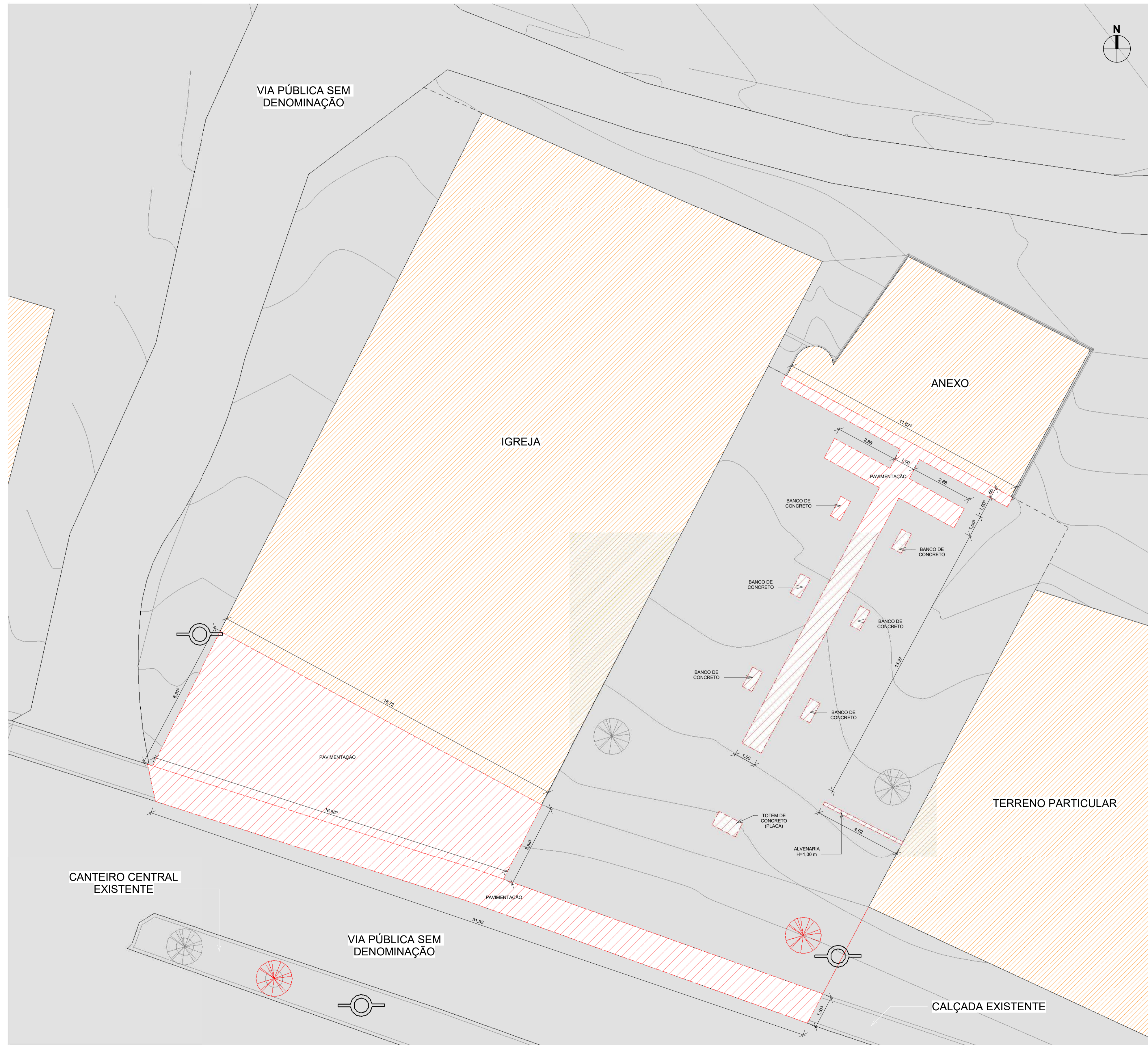
1 | PLANTA DE REFORMA 1 : 100
