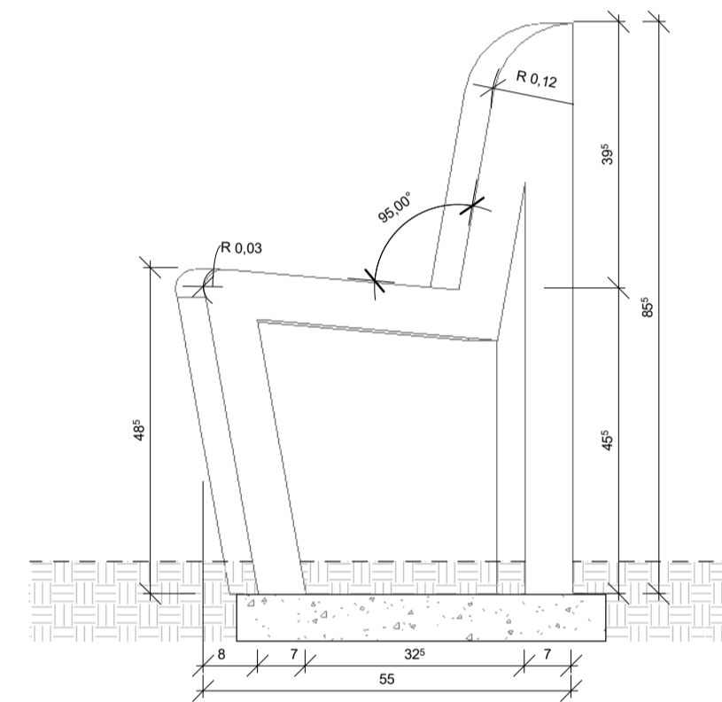
5 | CORTE - Banco de Concreto Curvo 05 1:10
