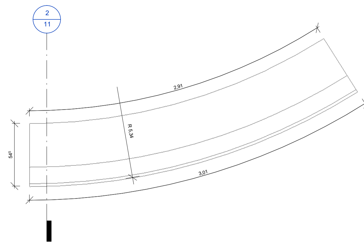
1 | PLANTA BAIXA - Banco de Concreto Curvo 04 1:20
