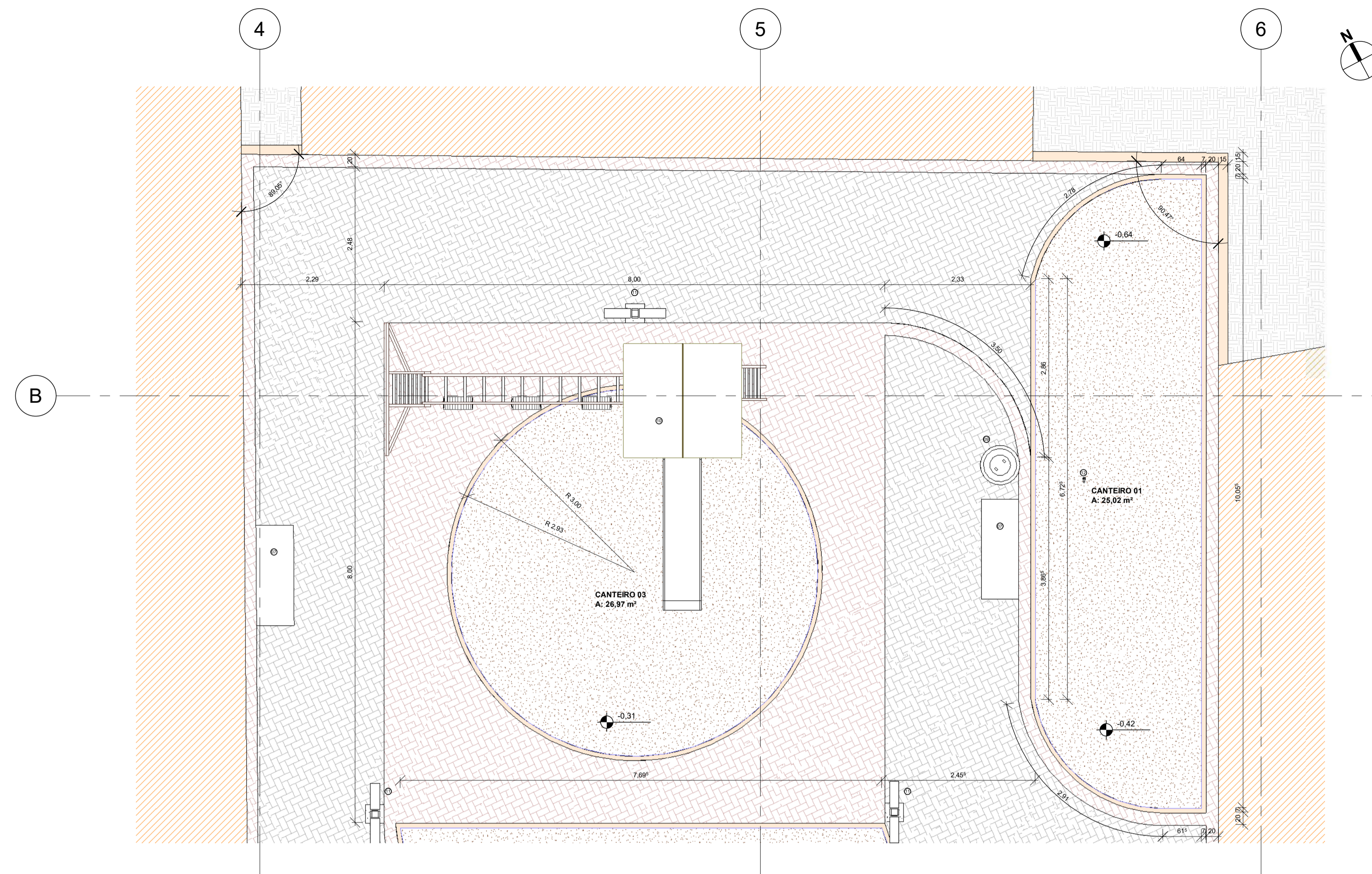
2 | PLANTA BAIXA - AMPLIAÇÃO TRECHO 06 1:50
