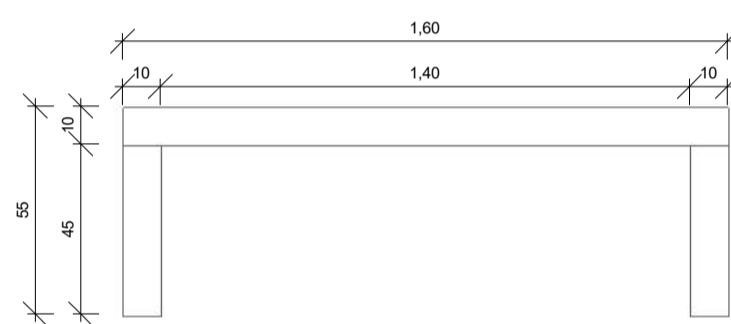
2 | VISTA - Banco de Concreto Reto 1 : 20
