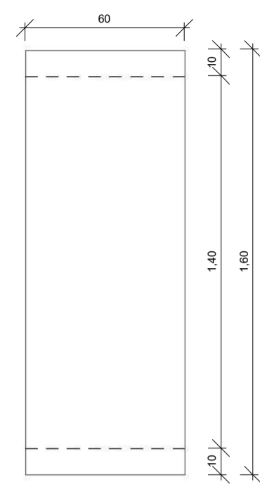
1 | PLANTA BAIXA - Banco de Concreto Reto 1 : 20
