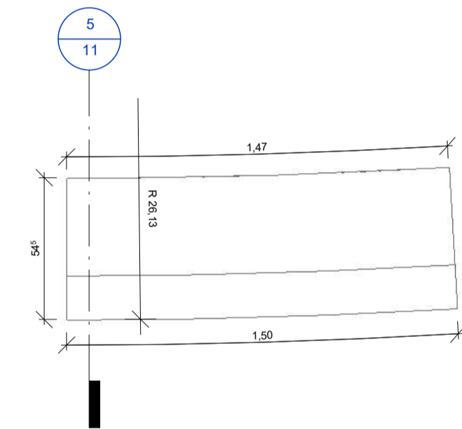
4 | PLANTA BAIXA - Banco de Concreto Curvo 05 1:20
