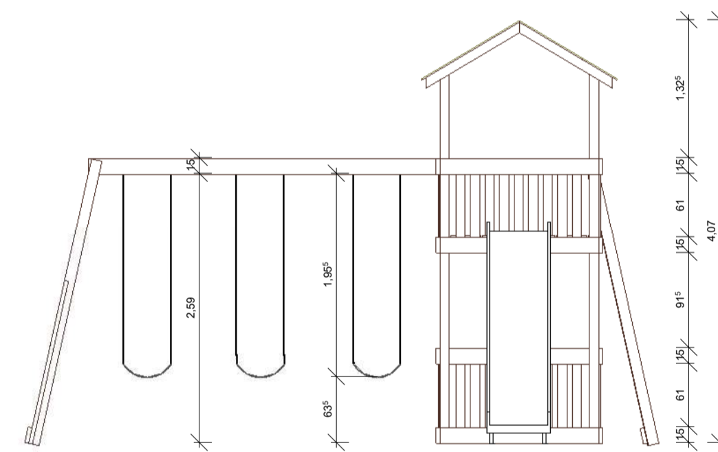
2 | VISTA 01 - Parque Infantil 1 : 50
