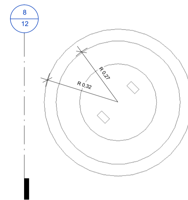
7 | PLANTA BAIXA - Lixeira de Concreto 1 : 10
