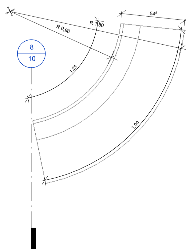
7 | PLANTA BAIXA - Banco de Concreto Curvo 03 1 : 20
