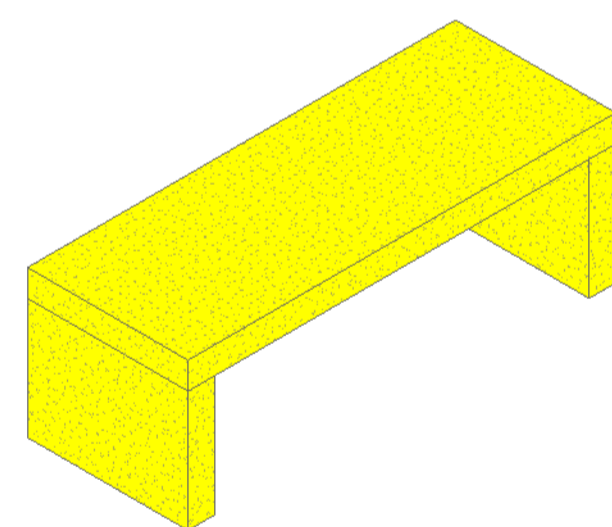
3 | PERSPECTIVA - Banco de Concreto Reto
