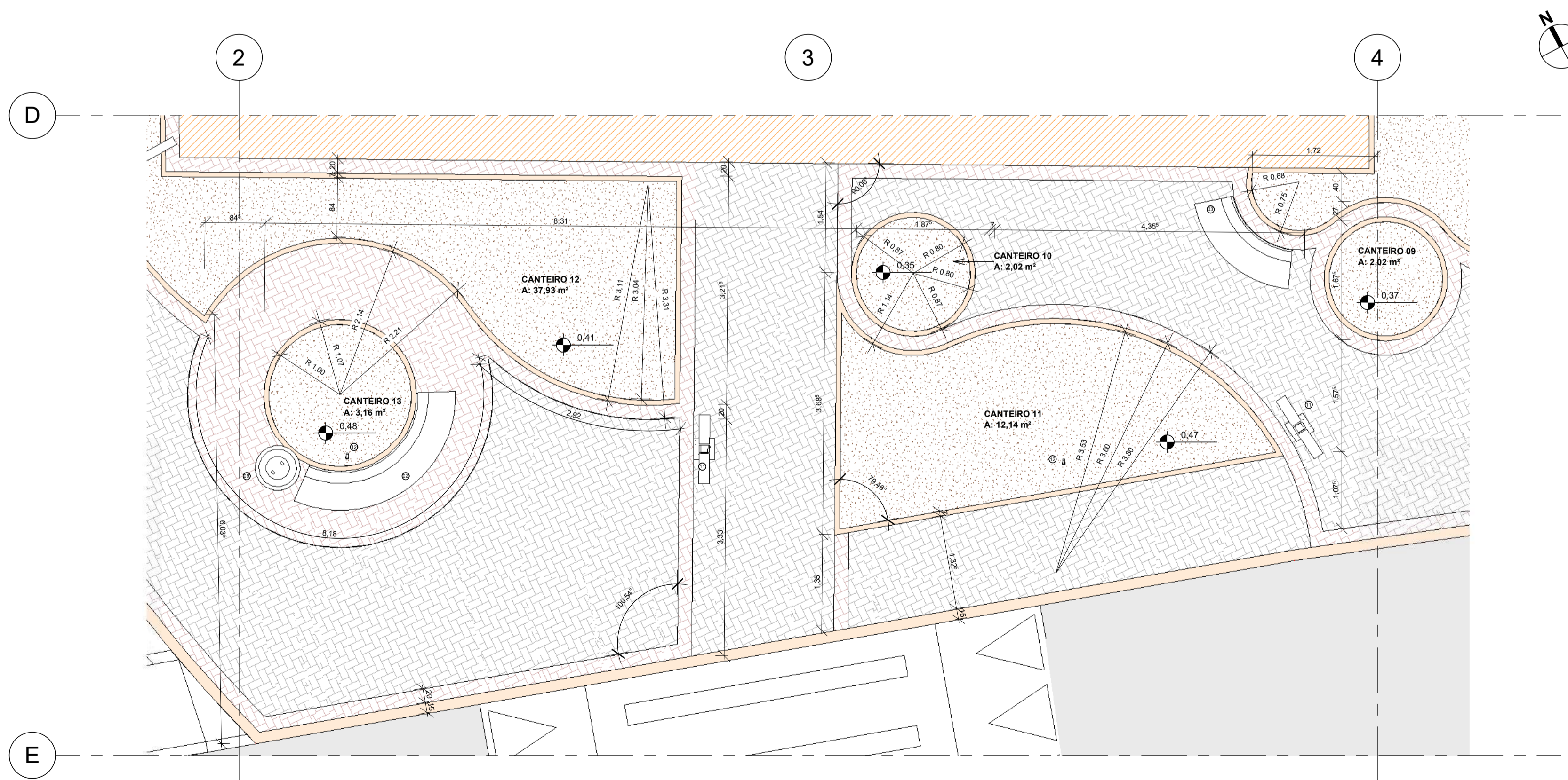
1 | PLANTA BAIXA - AMPLIAÇÃO TRECHO 03 1 : 50
