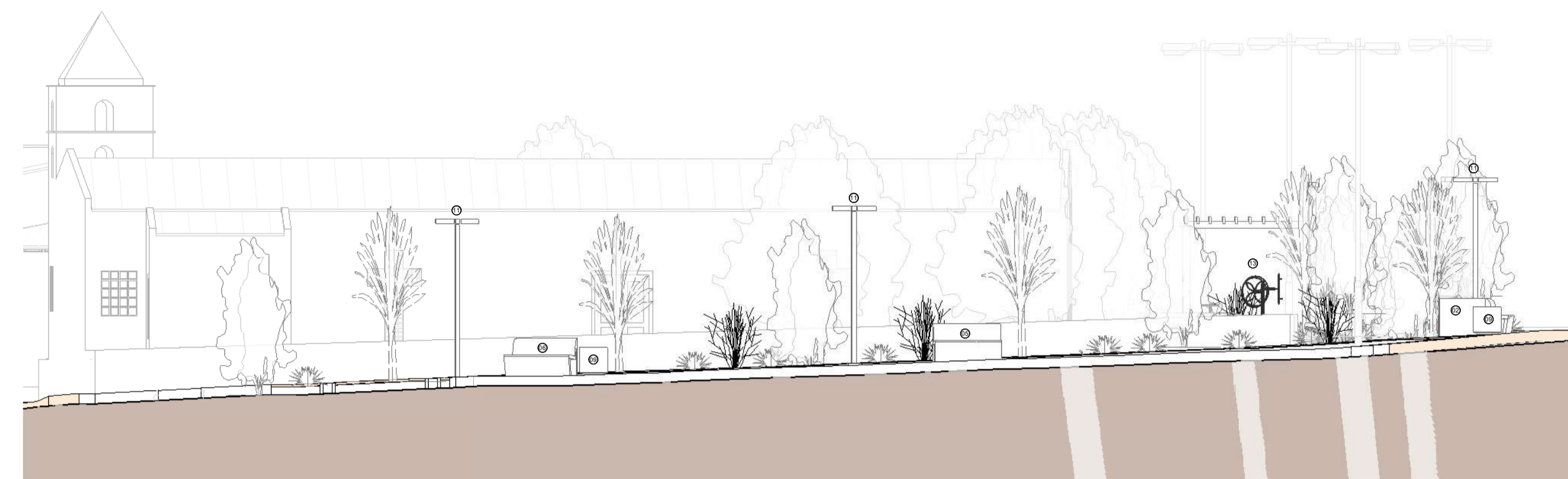
3 | Corte 03 1:100
