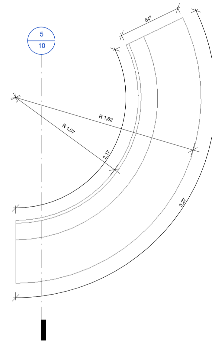
4 | PLANTA BAIXA - Banco de Concreto Curvo 02 1 : 20
