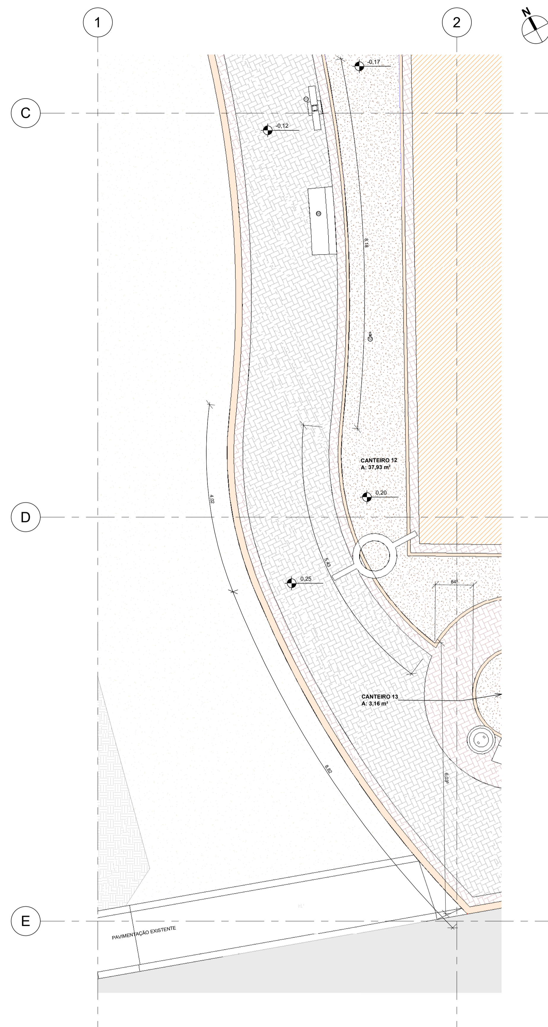
2 | PLANTA BAIXA - AMPLIAÇÃO TRECHO 02 1 : 50
