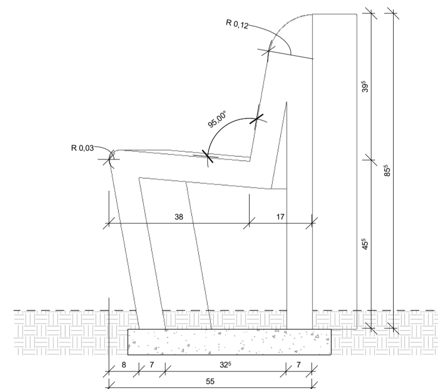
8 | CORTE - Banco de Concreto Curvo 06 1:10
