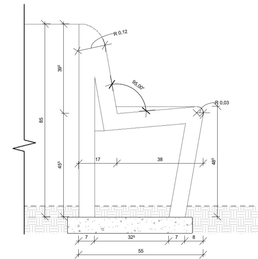
5 | CORTE - Banco de Concreto Curvo 02 1 : 10
