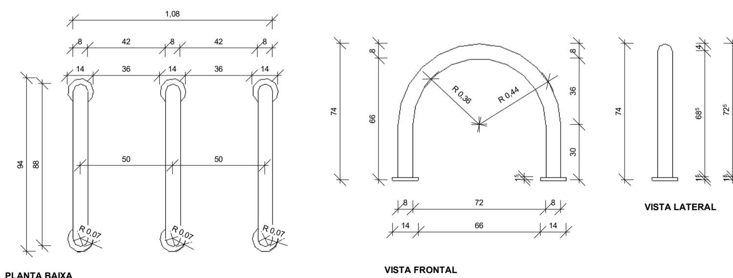
DET. BICICLETARIO EM AÇO 1 : 20
