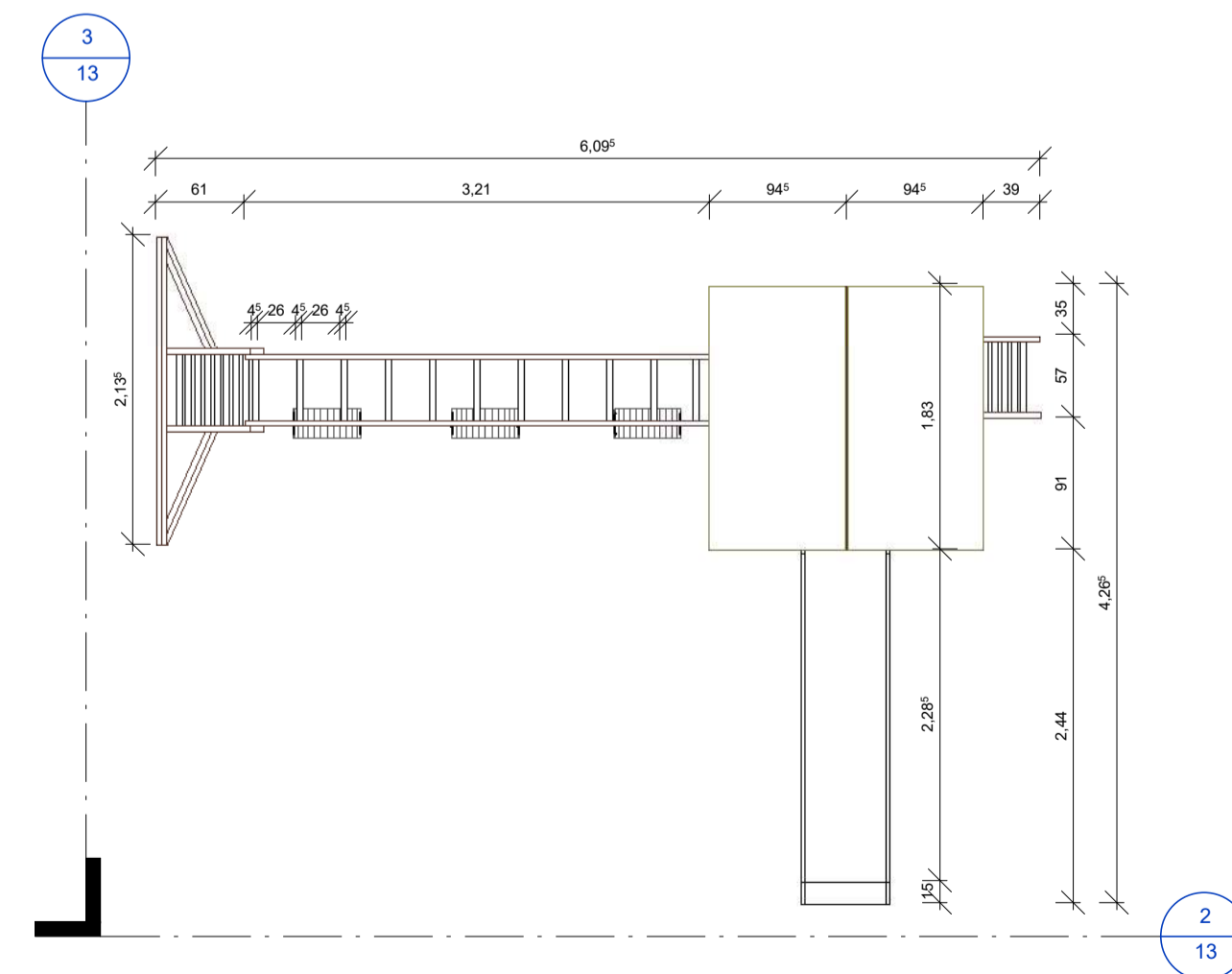
1 | PLANTA BAIXA - Parque Infantil 1 : 50
