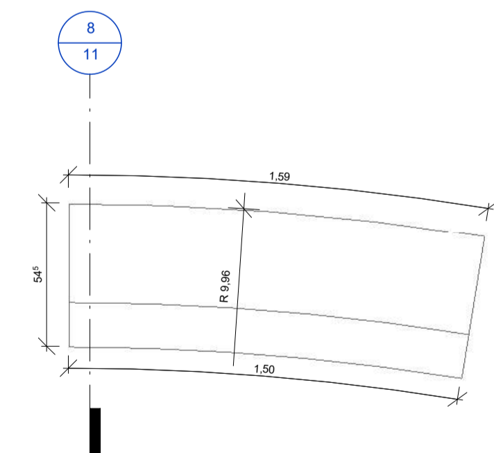
7 | PLANTA BAIXA - Banco de Concreto Curvo 06 1:20
