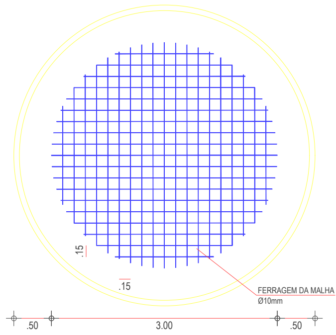
05 DETALHE DA ARMADURA DA FUNDAÇÃO ESC.: 1/50
