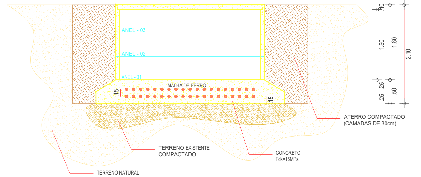
06 DETALHE DA FUNDAÇÃO ESC.: 1/50
