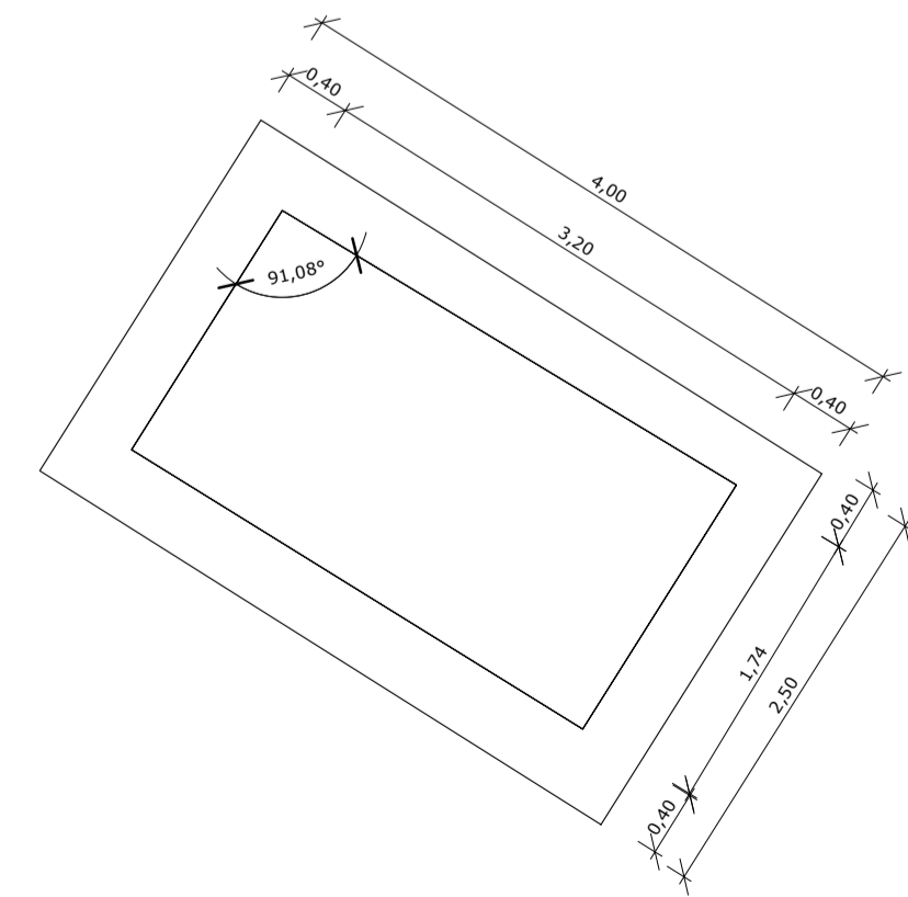
4 | DET. CANTEIRO 04 1 : 50
