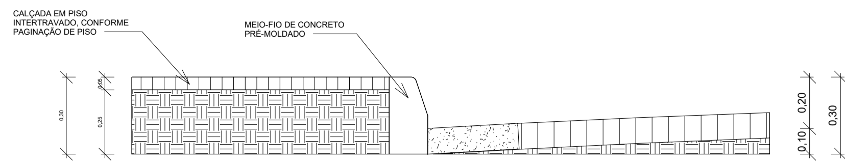
DET. MEIO-FIO 1:15
