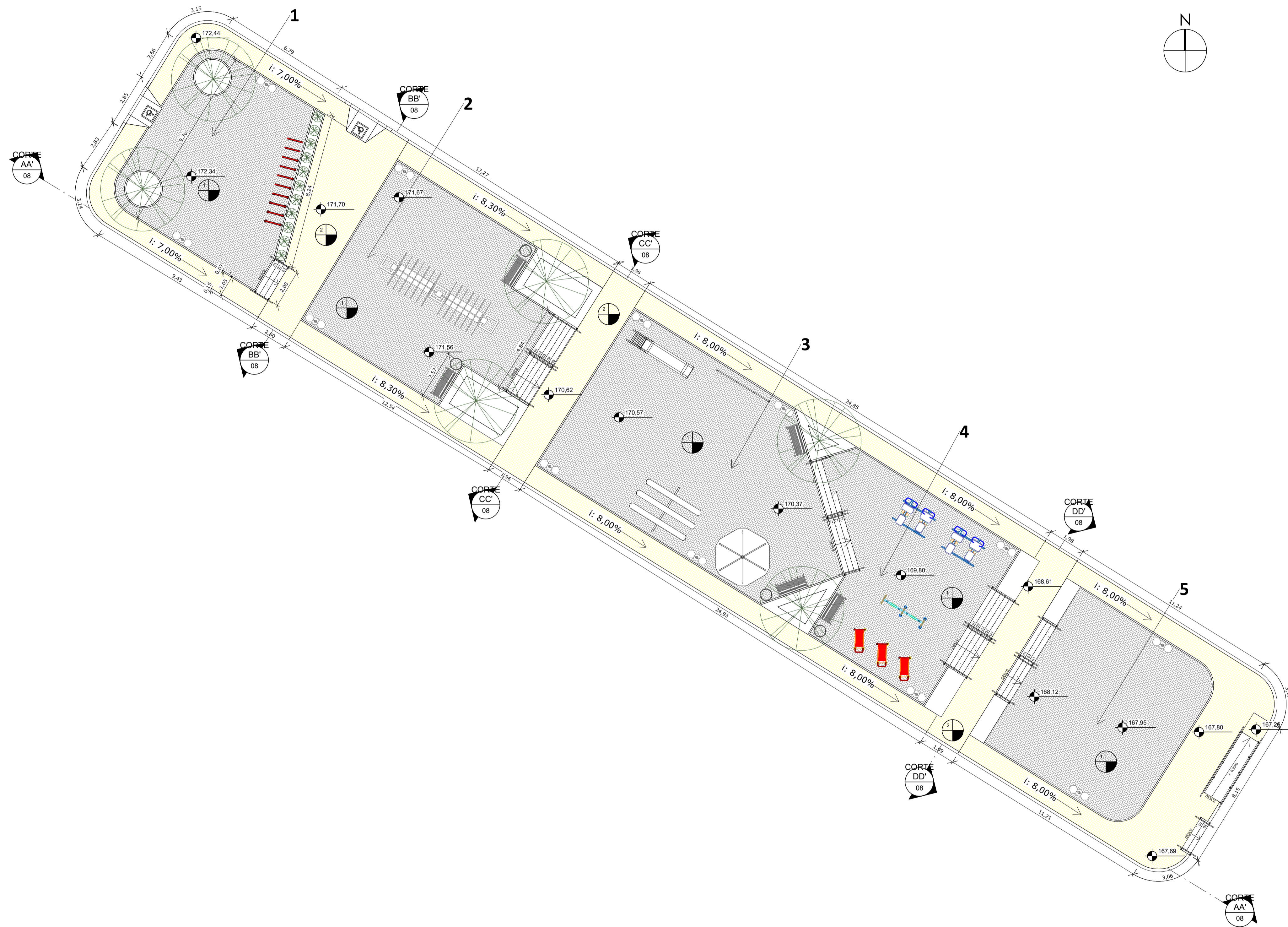
1 PLANTA BAIXA REFORMADA 1:125
