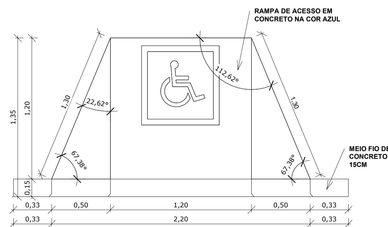
DET. DE RAMPA 1:20
