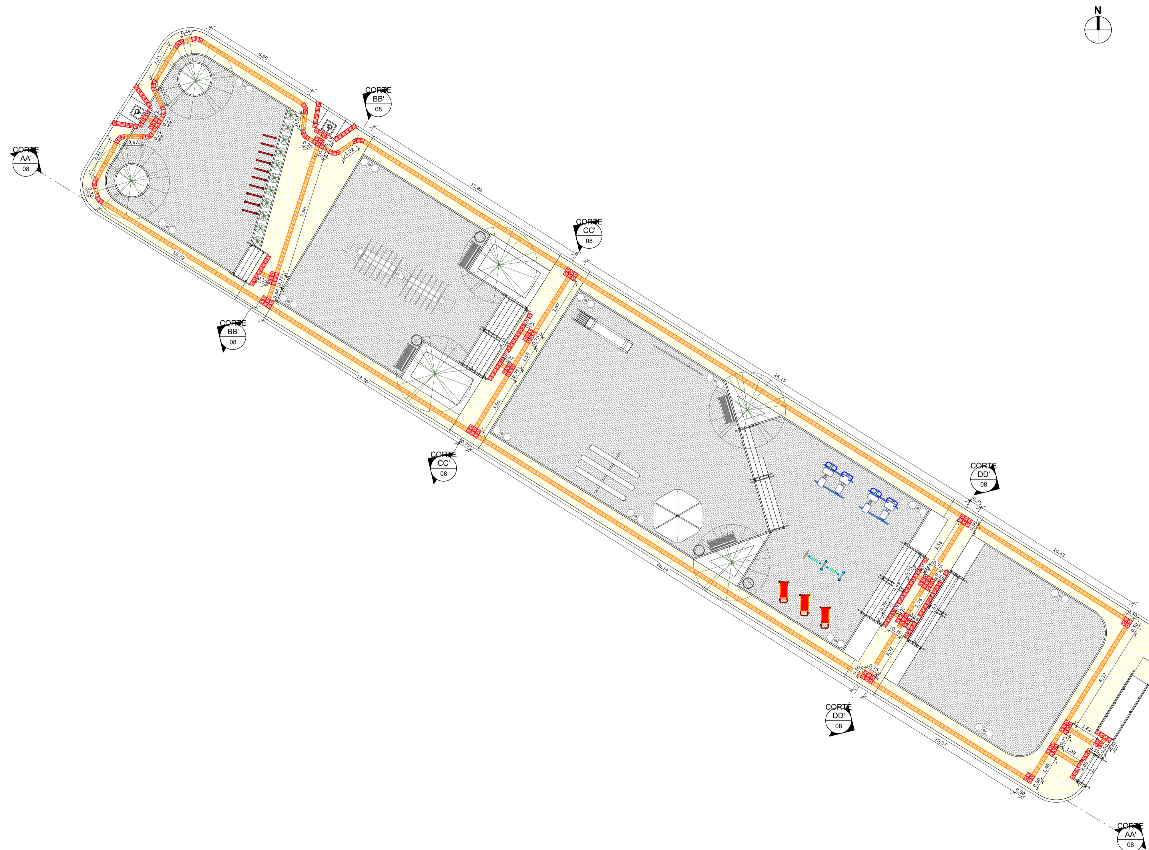
1 | PLANTA DE ACESSIBILIDADE 1 : 125
