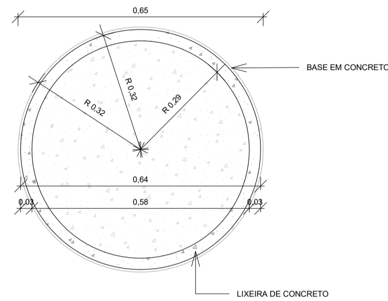
PLANTA BAIXA
