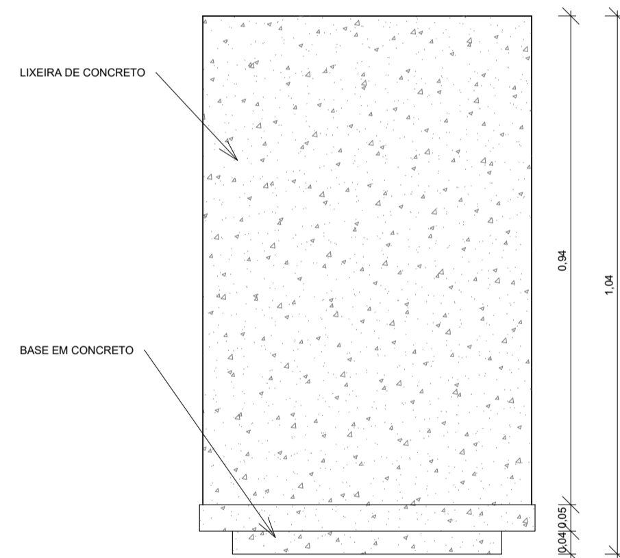
VISTA LATERAL
