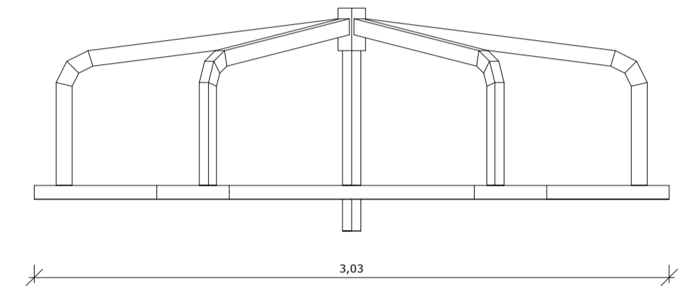
DET. GIRA GIRA 1 : 25
