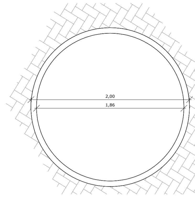
2 | DET. CANTEIRO 02 1 : 25
