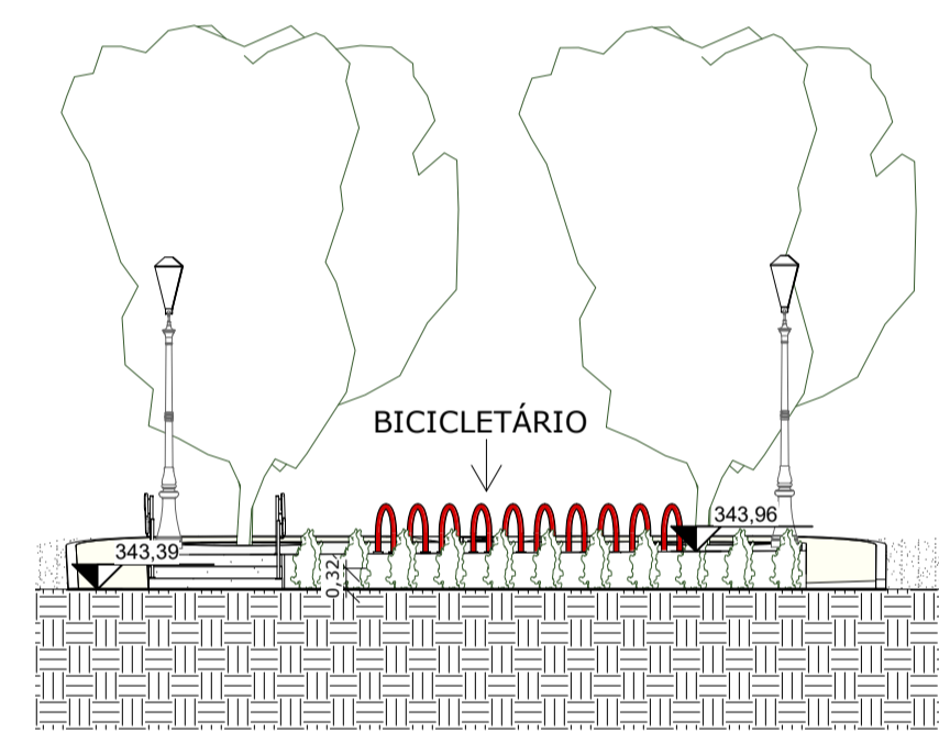
2 | CORTE BB' 1: 125
