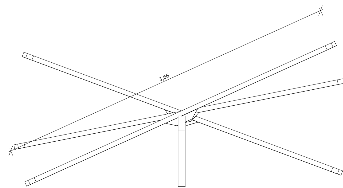
DET. GANGORRA 1 : 25
