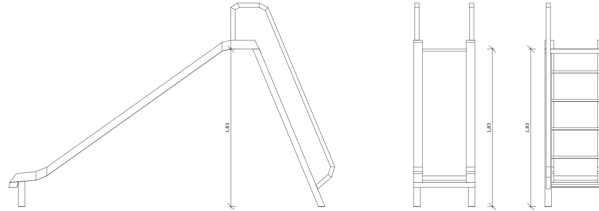
DET. ESCORREGADOR 1 : 25
