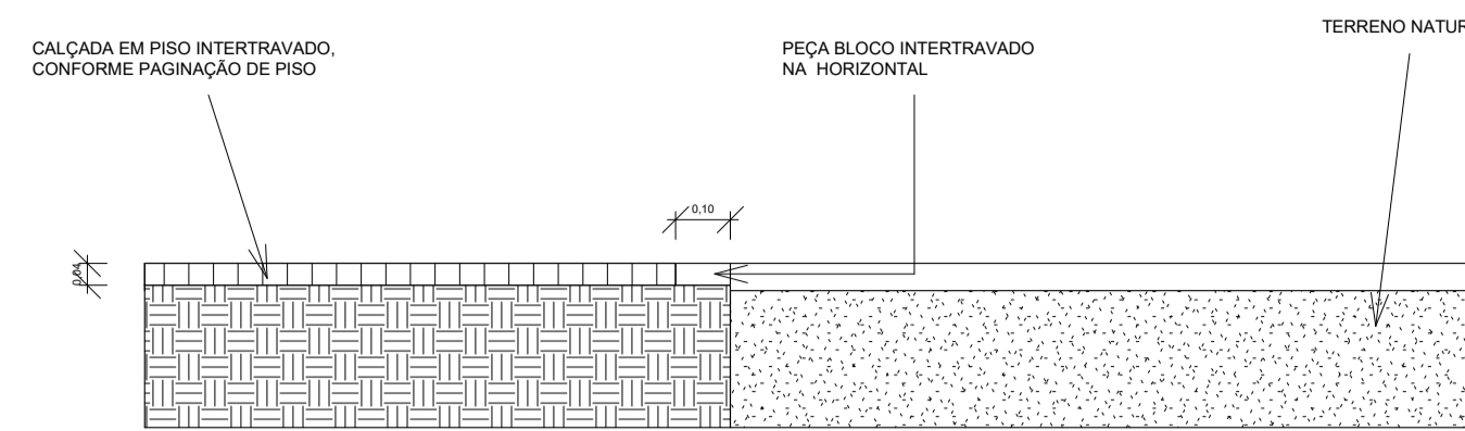
DET. ACABAMENTO DE PISO 1:15
