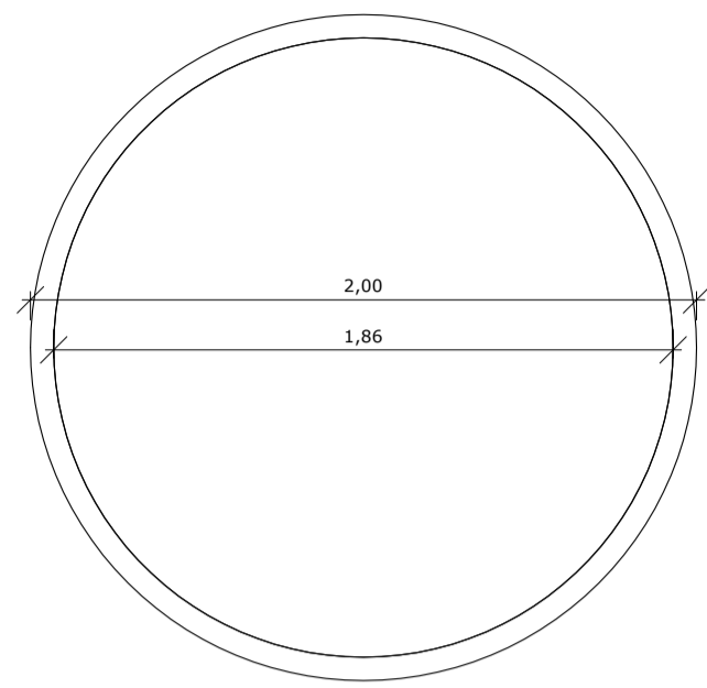
1 | DET. CANTEIRO 01 1 : 25
