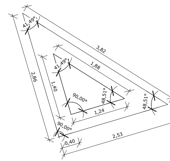
5 | DET. CANTEIRO 05 1 : 50
