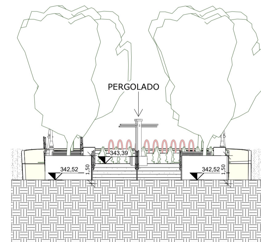
3 | CORTE CC' 1: 125
