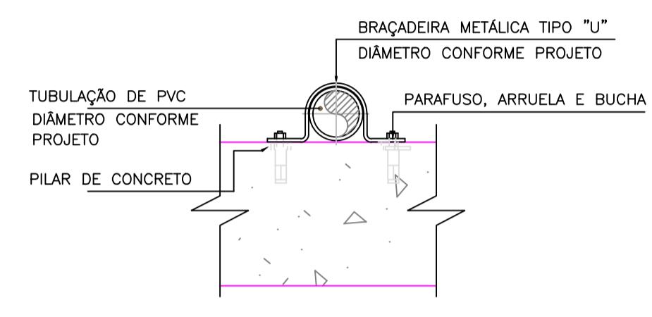
04 DETALHE DA FIXAÇÃO DE DESCIDAS SEM ESCALA
