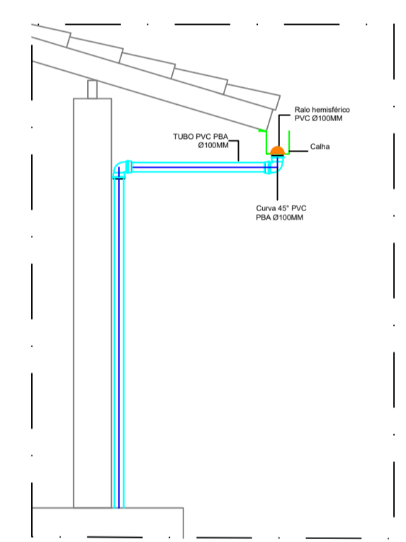
05 DETALHE DO RALO SEM ESCALA
