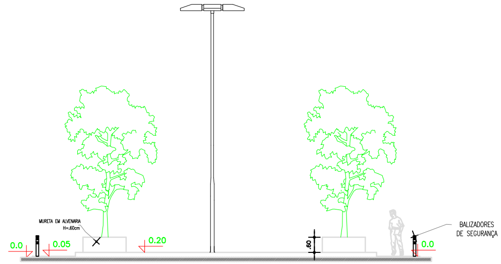
○ CORTE BB 1/150
