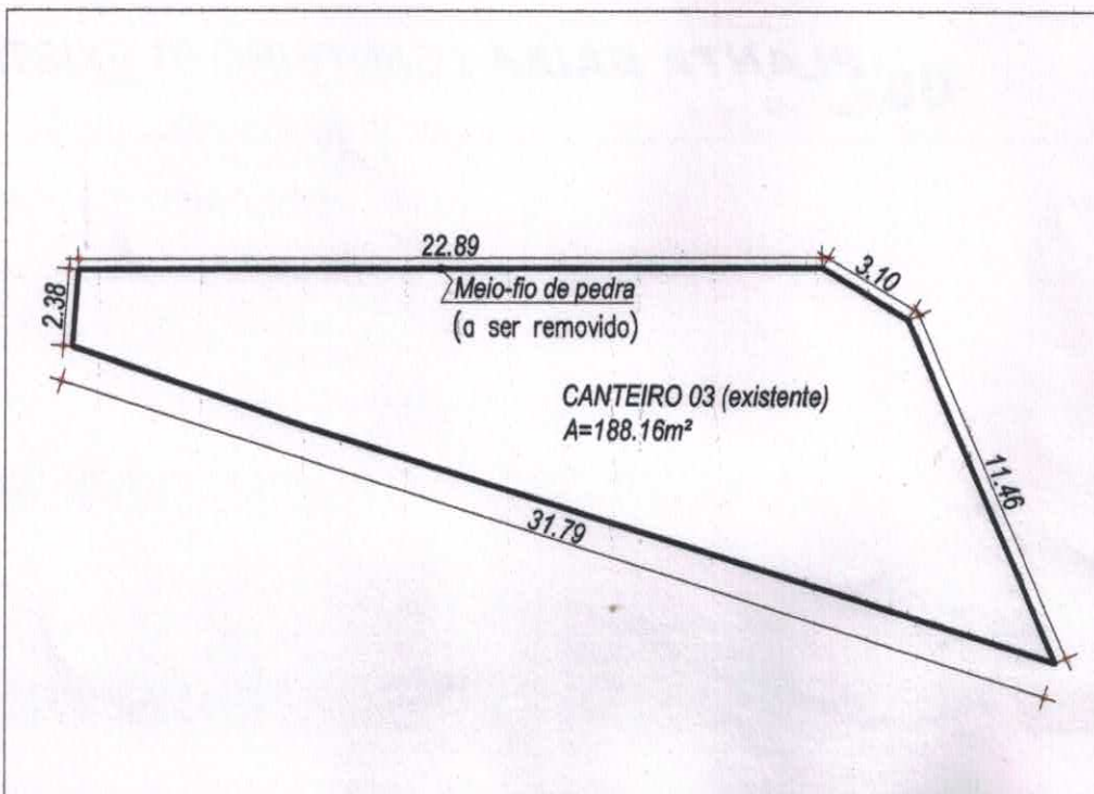
11 PLANTA BAIXA (CANTEIRO 03 EXISTENTE) esc 1:250
